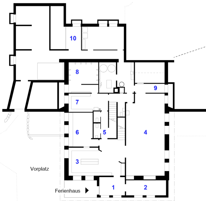
Untergeschoss
