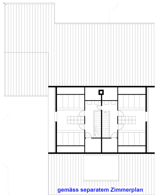
Dachgeschoss
